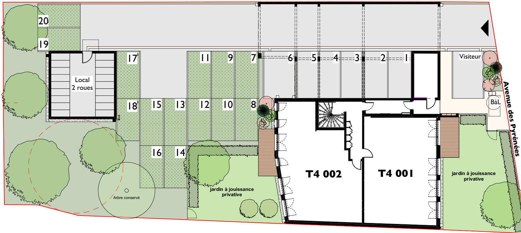
PLAN SYNOPTIQUE - REZ-DE-CHAUSSEE
